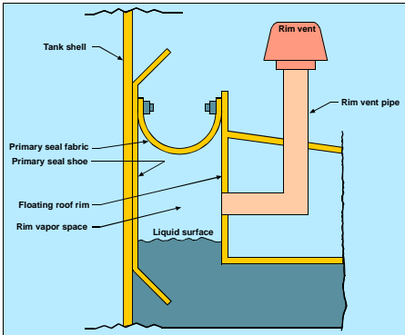
Rim Vent
